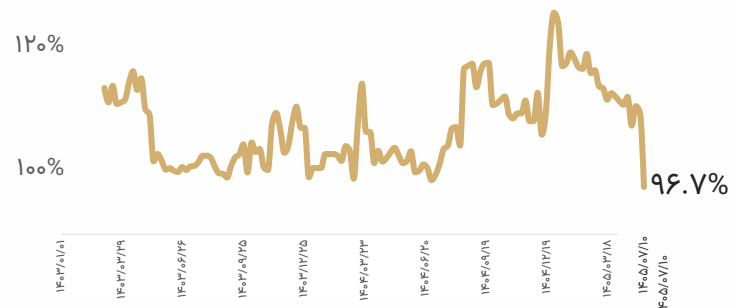
نسبت ورق گرم به اسلب
