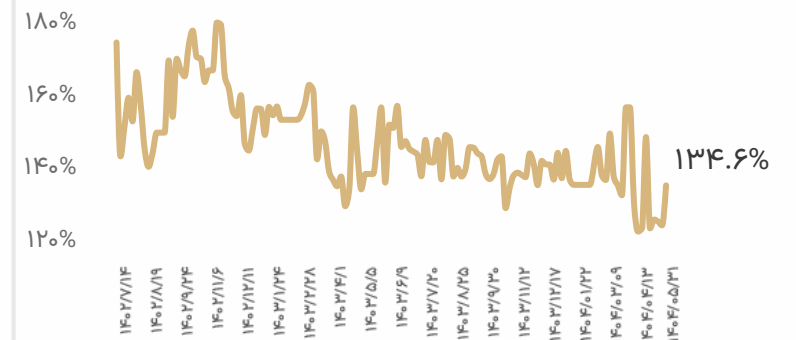
نسبت ورق گالوانیزه به اسلب
